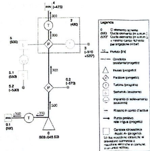
Diga di Casalbuono - Schema idrico - Alternativa 1 Funzionamento invernale (stagione non irrigua, 7 mesi)
