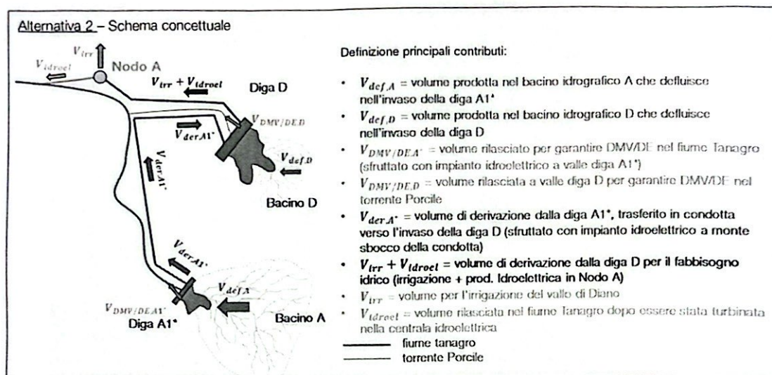
Figura 2-1: Alternativa 2 (A1*+D), schema concettuale di funzionamento (fonte DOCFAP, 2024)
