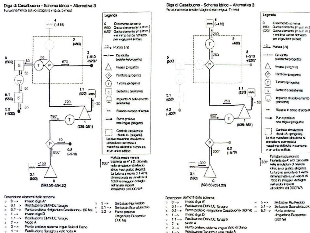
Figura 3-2: Alternativa 3 (A2*+D), schemi irrigui nelle stagioni estiva (sinistra) e invernale (destra) (fonte DOCFAP, 2024)
