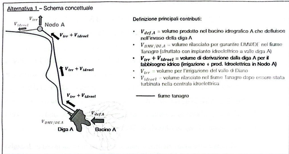
Figura 1-1: Alternativa 1 (A), schema concettuale di funzionamento (fonte DOCFAP, 2024)
