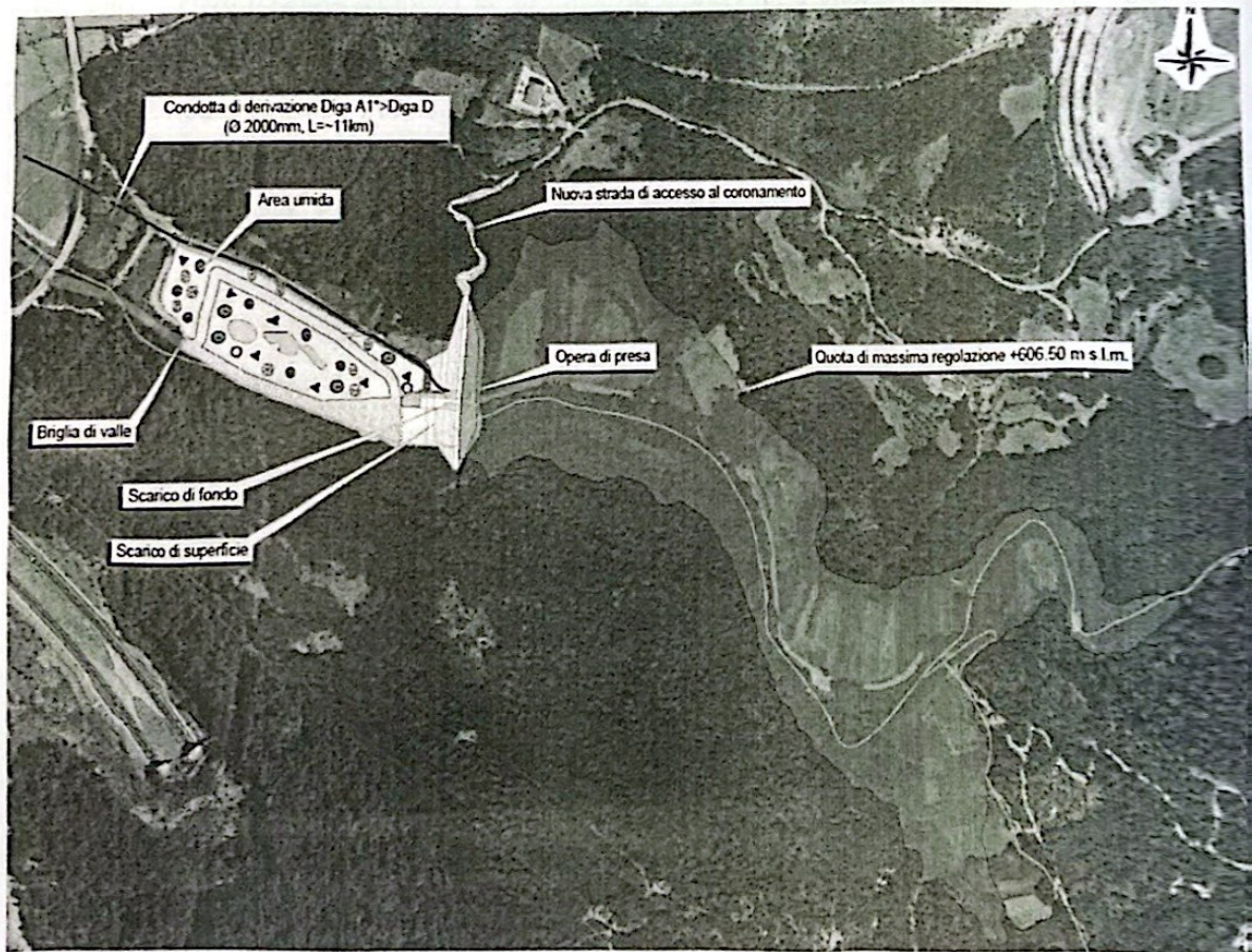
Figura 1-3: Alternativa 1 (A), planimetria generale di progetto sito A (fonte DOCFAP, 2024)
