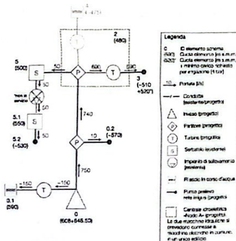
Diga di Casalbuono - Schema idrico - Alternativa 1 Funzionamento estivo (stagione irrigua, 5 mesi)
